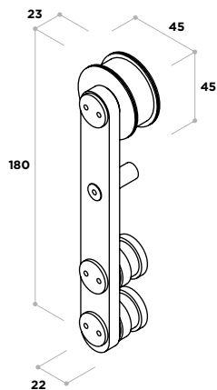
02010052 Tope guía Alter Acero inoxidable
