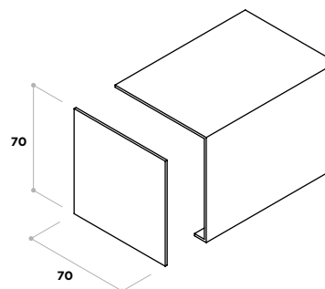
02030155 Forro acero inox. guía Muse Acero inoxidable
