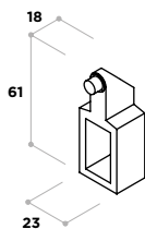
02010052 Tope guía Alter Acero inoxidable
