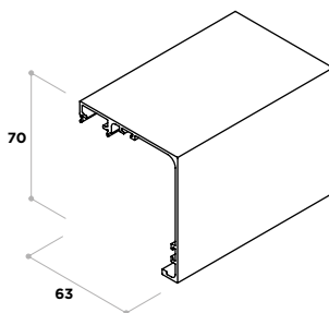
02030277 Forro aluminio guía Muse Aluminio
