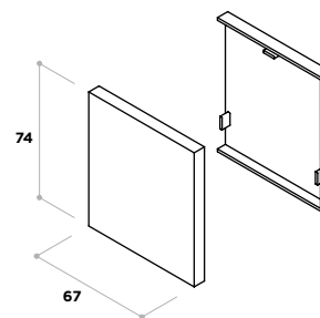
02010464 Juego tapetas forro Muse Aluminio
